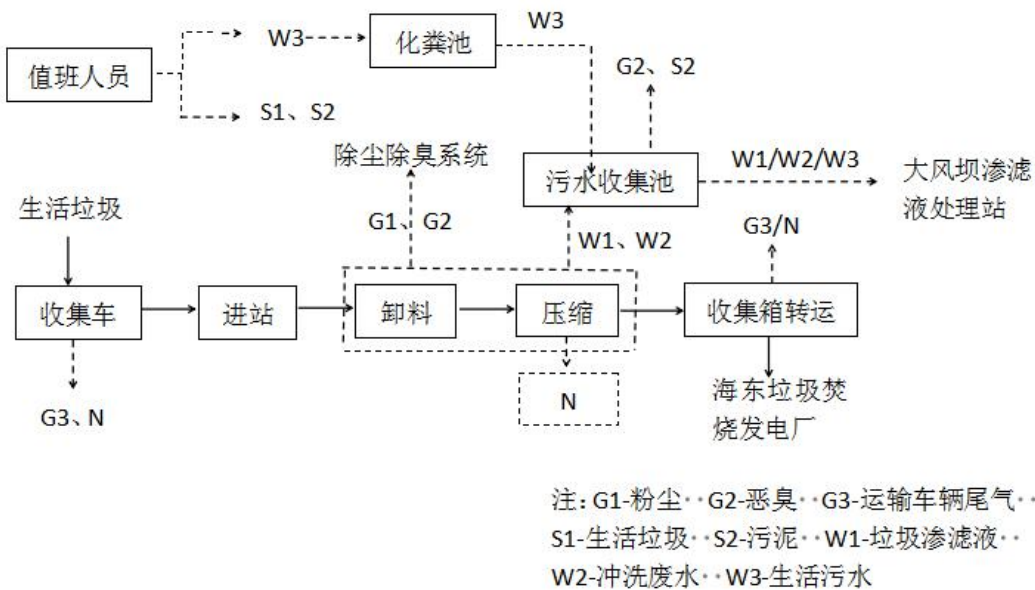
图 3-1 项目工艺流程及产污环节
