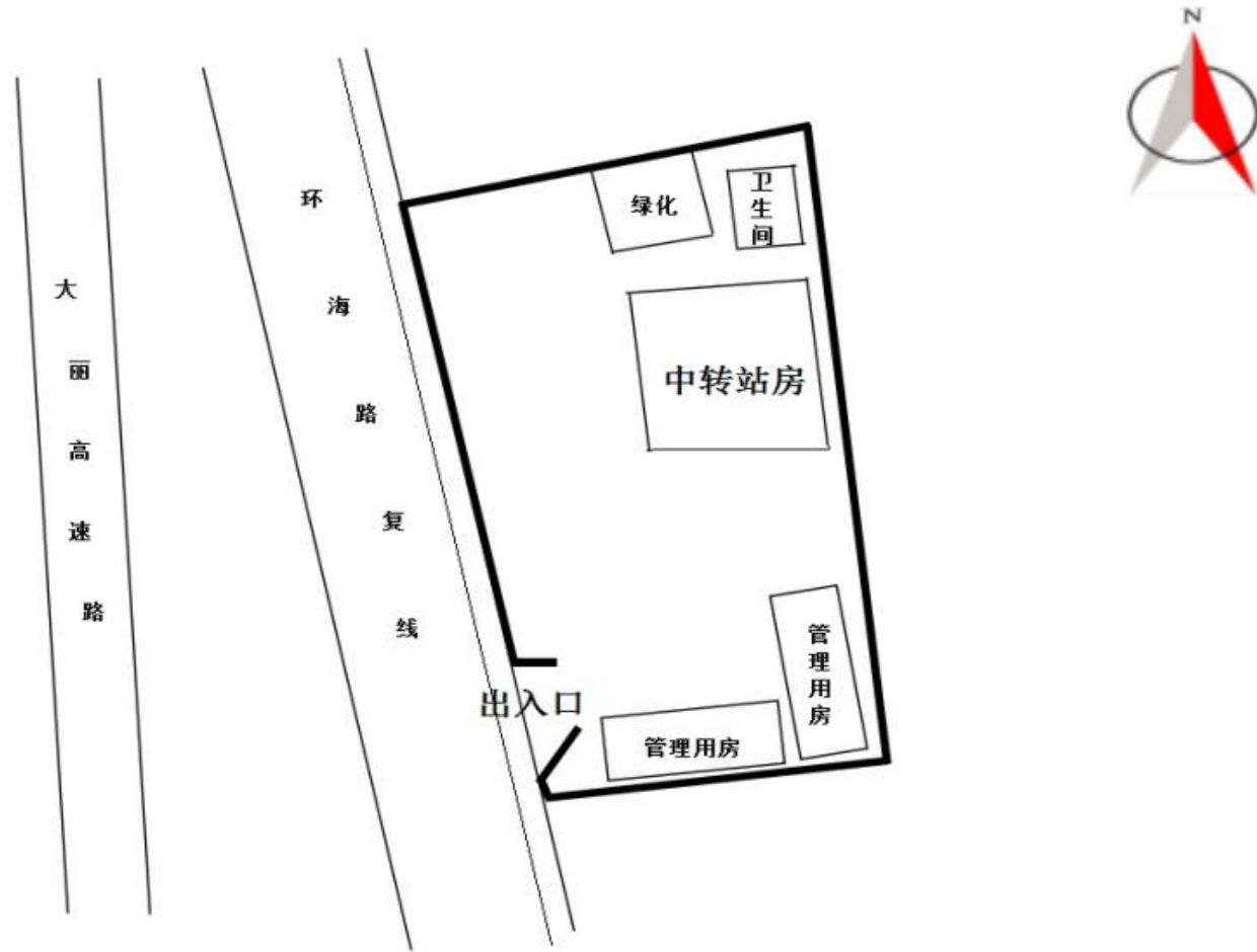
项目平面布置简图
