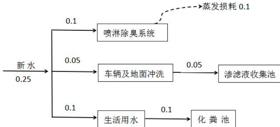
图 3-3 项目水平衡图 单位：m 3 /d
